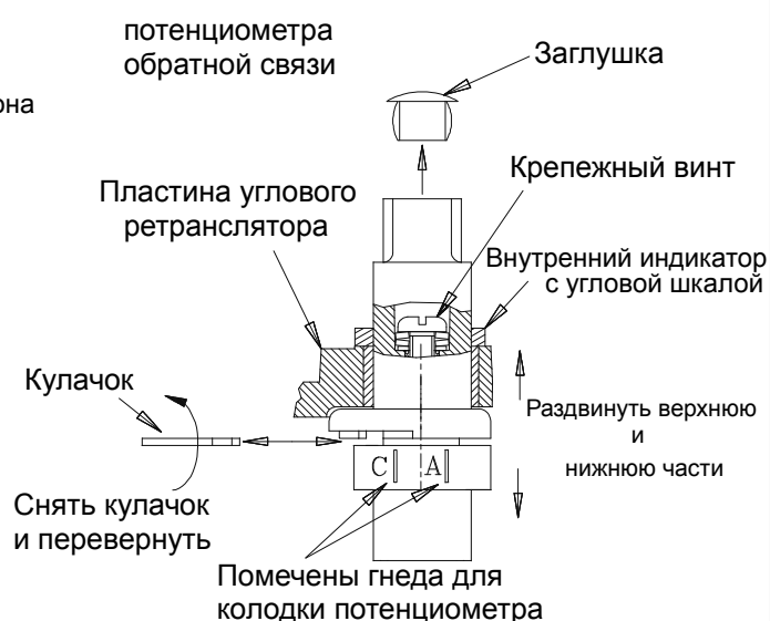
РИСУНОК 8. МУФТА – СМЕНА ВРУЧНУЮ
